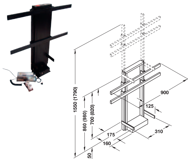
Hebesystem
