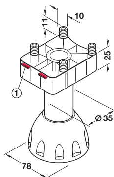
Bohrbild
