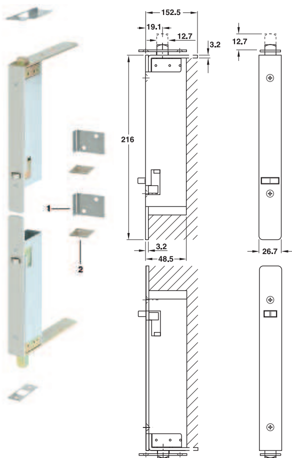
1 Auflaufplatte 2 Unterlegplatte
