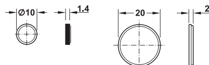
Magnetscheibe
