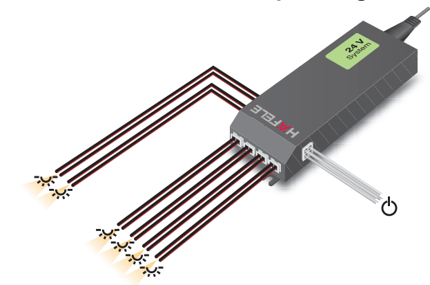
Parallelschaltung
