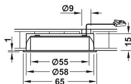
Einbaumontage
