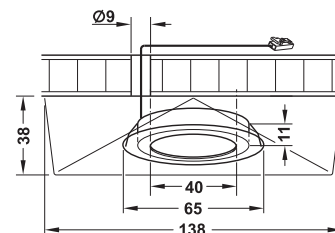
Unterbaumontage mit Dreieck-Gehäuse
