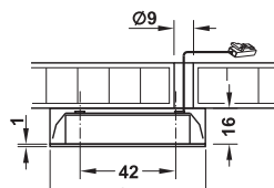
Unterbaumontage mit Ring
