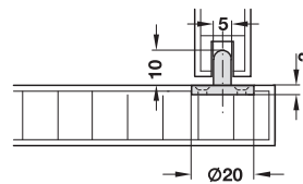
Einfach-Führung zum Schrauben und Einpressen in eine Bohrung
