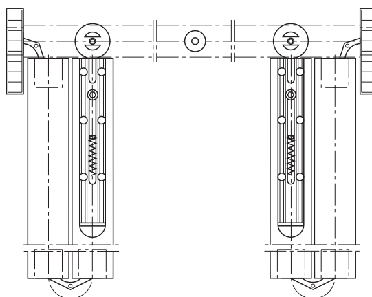
4-flügelige (2+2-flügelige) Falttür
