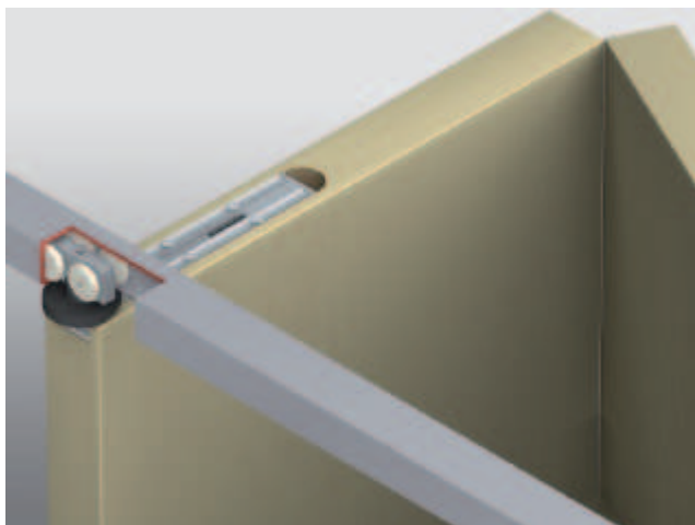
2-flügelige Falttür geschlossen
