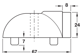
Bodentürpuffer TZ 5000
