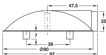
Fußplatte TZ 55, TZ 56
