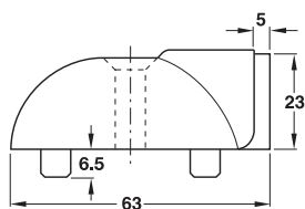
Bodentürpuffer
