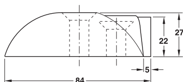
Bodentürpuffer
