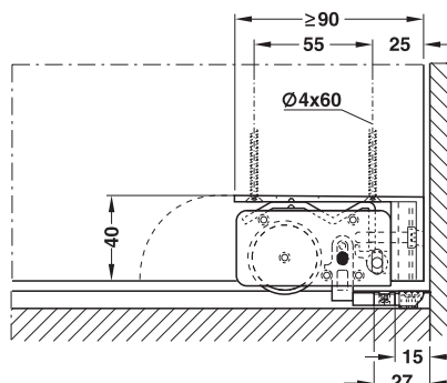
Schnitt Rollenwagen und Bodenführung
