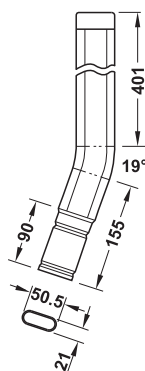
Montage an Einhängelleiter
