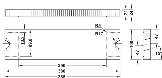
Stufen für Holzstufenleiter
