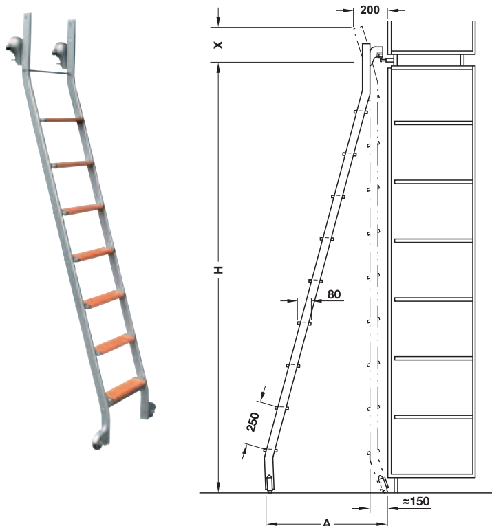
Rollbeschlag oben
