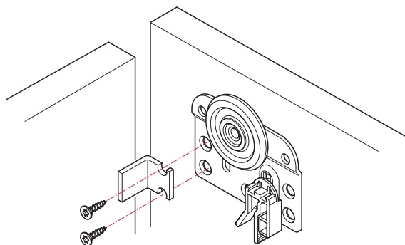
Befestigung des Mitnehmerwinkels
