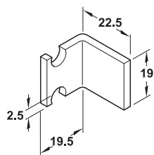
Winkel für innere Tür
