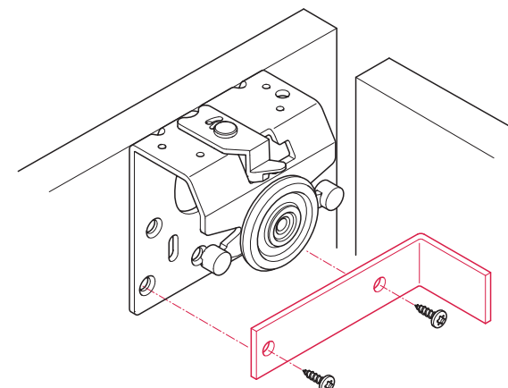
Winkel für äußere Tür
