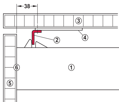
Mitnehmerwinkel montiert
