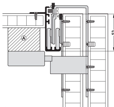
Ⓐ Zwischenplatte
